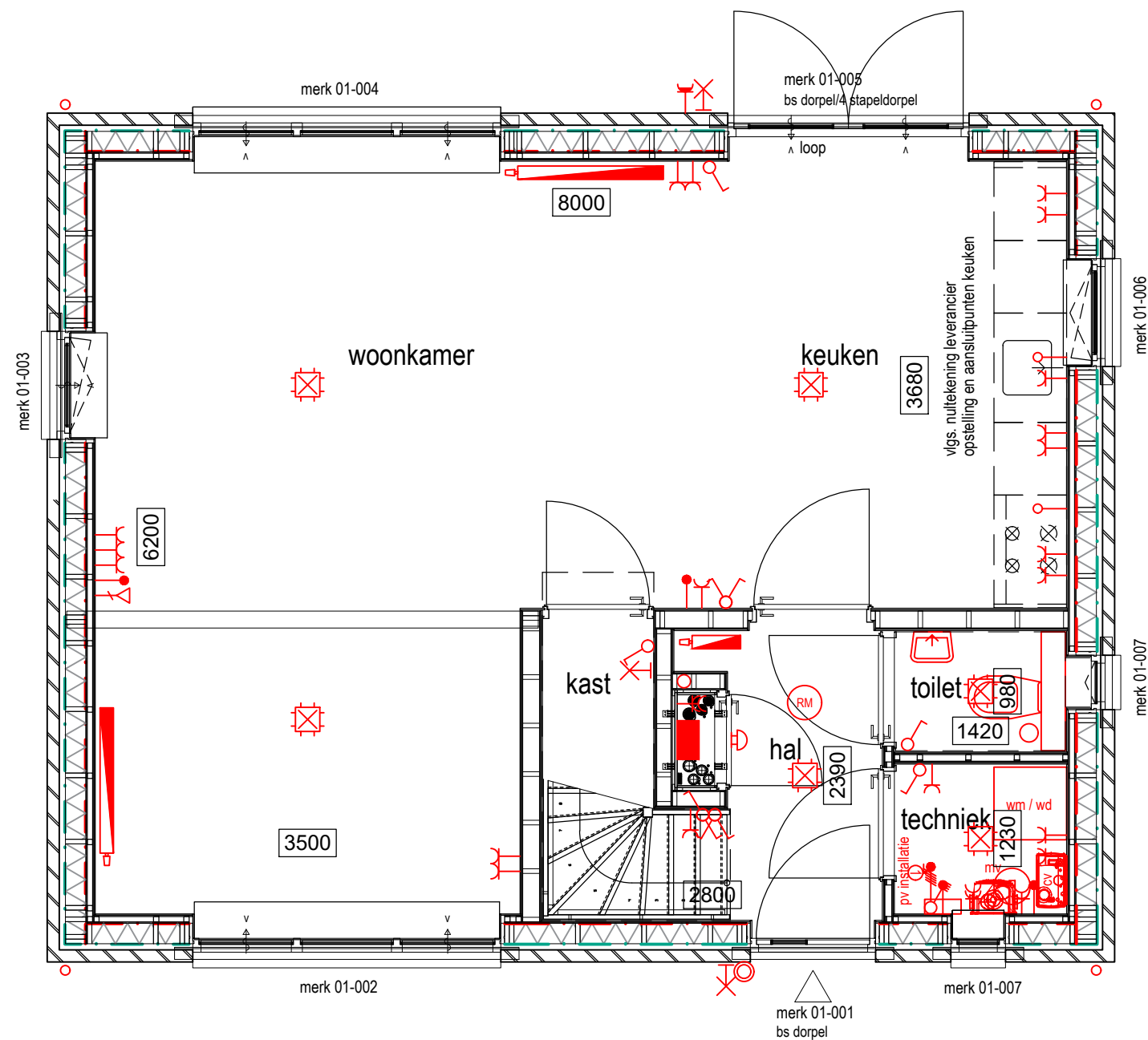
verkooptekening basiswoning kavel 01 (BEGANE GROND)
